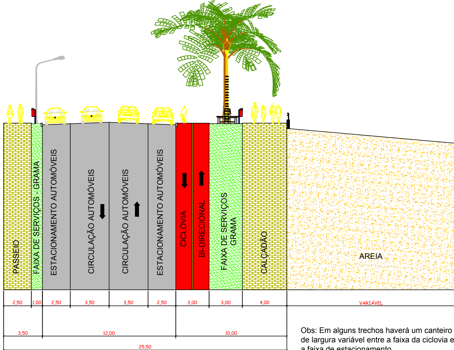
Gabarito da Rua Zimmer Escala 1:200
