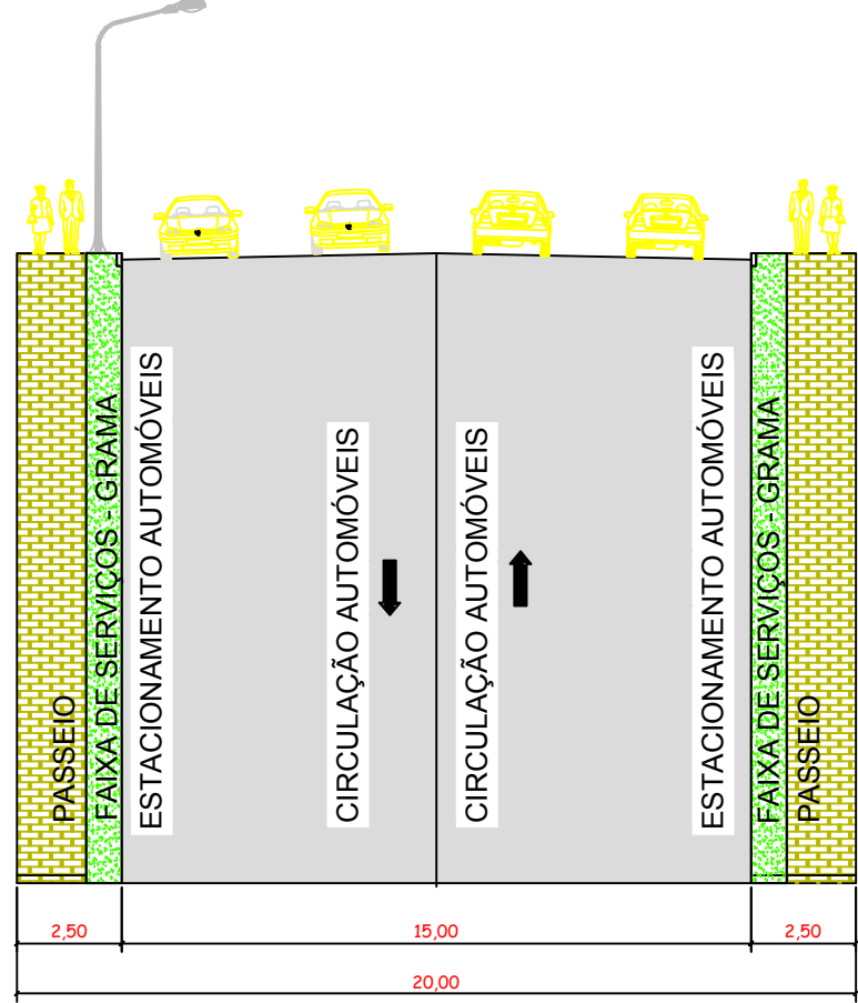
Gabarito da Rua Júlio Schwengber Sobrinho Escala 1:200
